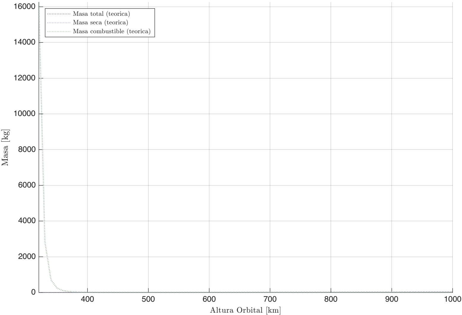
Desglose de Masas vs. Altura Config: 1 Sat, 1 Tel, Det 2, Cassegrain
